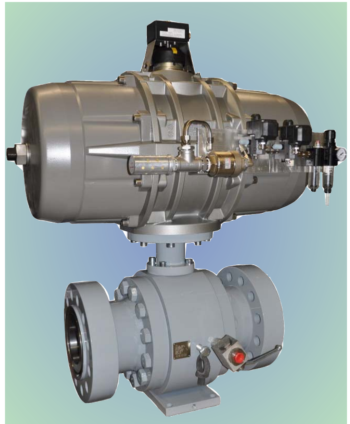
Kugelhahn 6" ANSI 1500lbs mit Steuerung ball valve 6" ANSI 1500lbs with control unit
