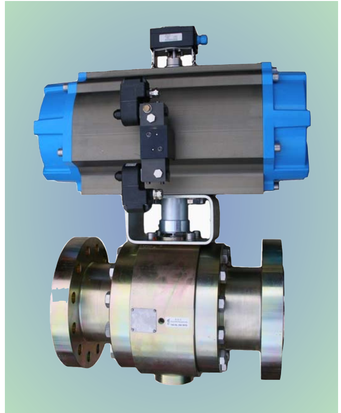
metallisch dichtender ASC KH 6" mit Antrieb metall seat ASC ball valve 6" with actuator
