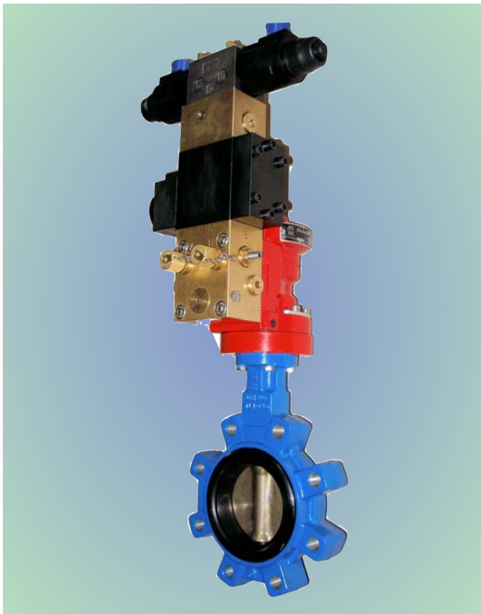
Absperrklappe mit hydraul. Antrieb + Steuerung butterfly valve with hydr. actuator + controlunit
