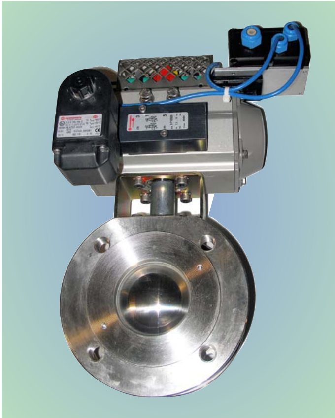
Kompakt Kugelhahn ATEX mit Anschlußbox wafer ball valve ATEX with connecting box
