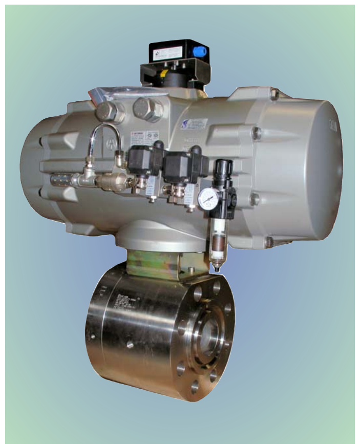
metallisch dichtender ASC KH 4" ANSI 2500lbs metall seat ASC ball valve 4" ANSI 2500lbs
